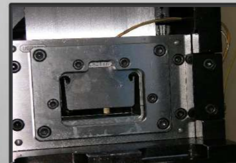
Cutting die
